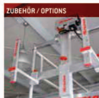
HWT elektrisches Material-Transport-System für Rollgerüste, ideal für Montage- und Installationsarbeiten in der Höhe, bei maximaler Sicherheit. Weitere Informationen auf Seite 89 HWT Système de montée des matériaux électrique pour échafaudages mobiles, idéal pour des travaux de montage et d'installation, en toute sécurité. Plus d'informations à la page 89
